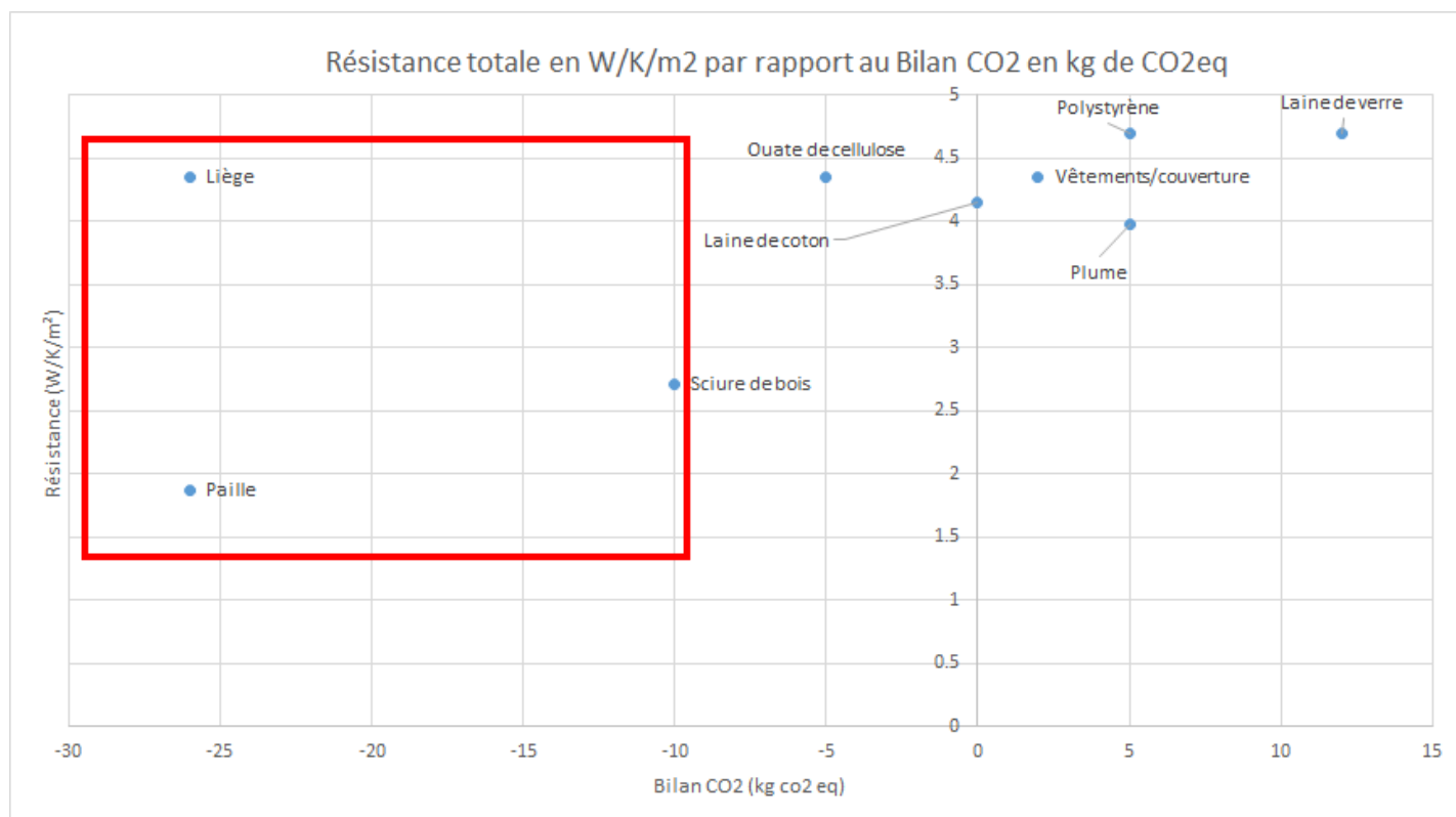
Figure 5 : Comparaison performance thermique/bilan CO 2 de différents isolants [5]
