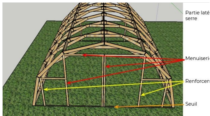
Tunnel de 4.2m par 4.8m
