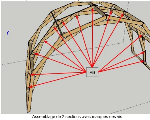
Assemblage de 2 sections avec marques des vis
