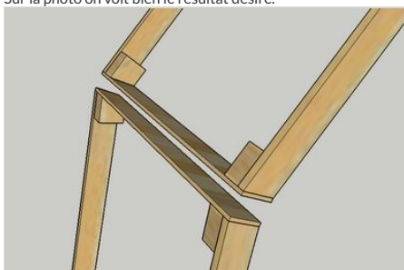
Assemblage de deux modules
