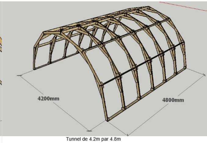
Tunnel de 4.2m par 4.8m
